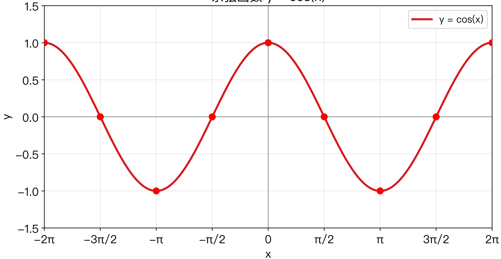
余弦函数 y = \cos(x)
