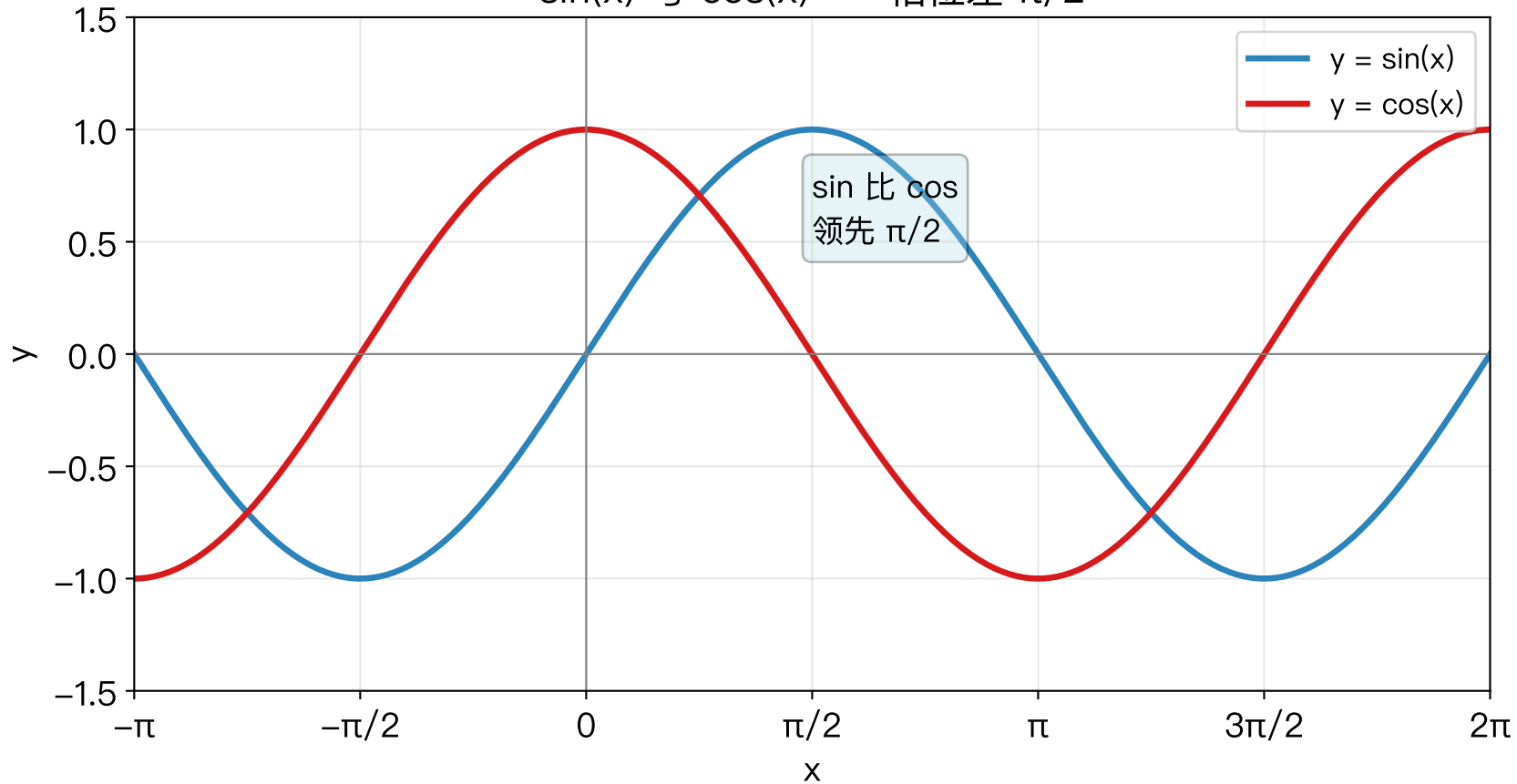
\sin(x) 与 \cos(x) ——相位差 \pi/2
