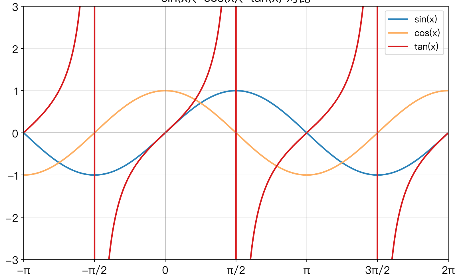
\sin(x) 、 \cos(x) 、 \tan(x) 对比
