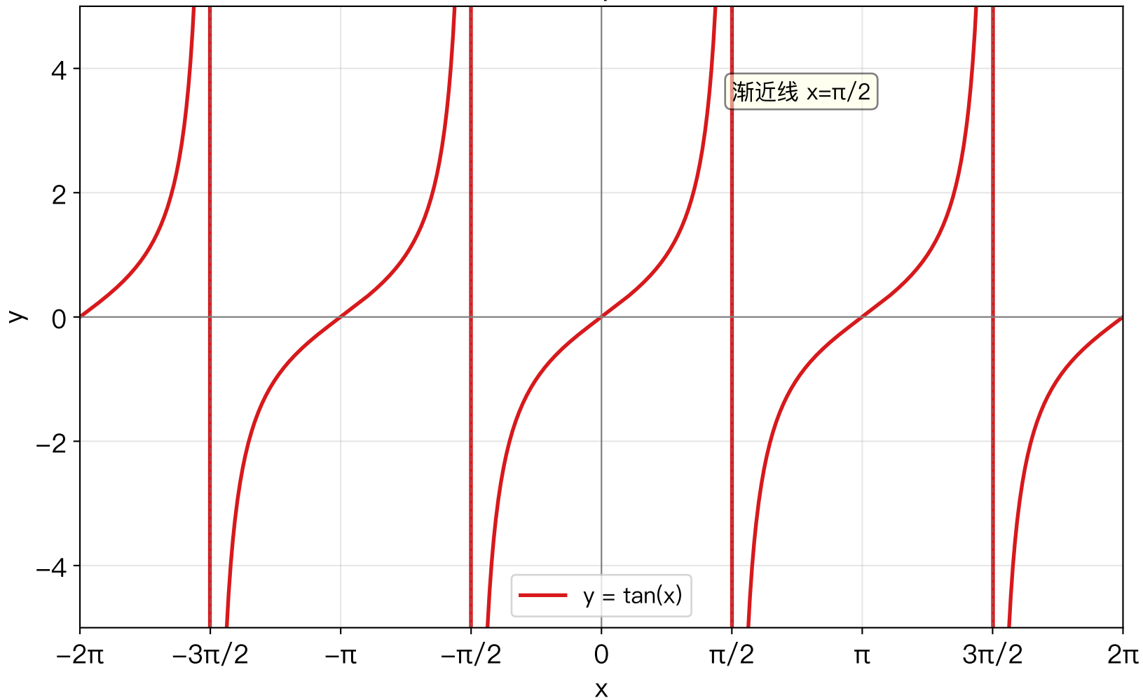
正切函数 y = \tan(x)
