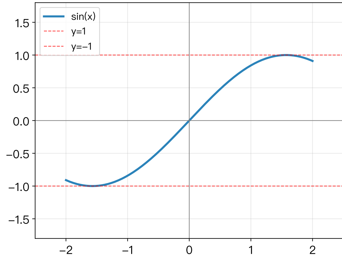
有界函数 —— |\sin(x)| \leq 1
