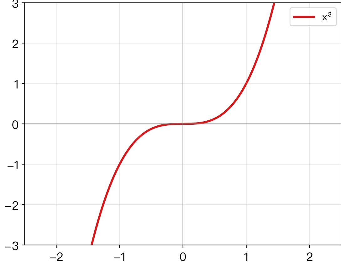
无界函数 —— x^3 无上下界
