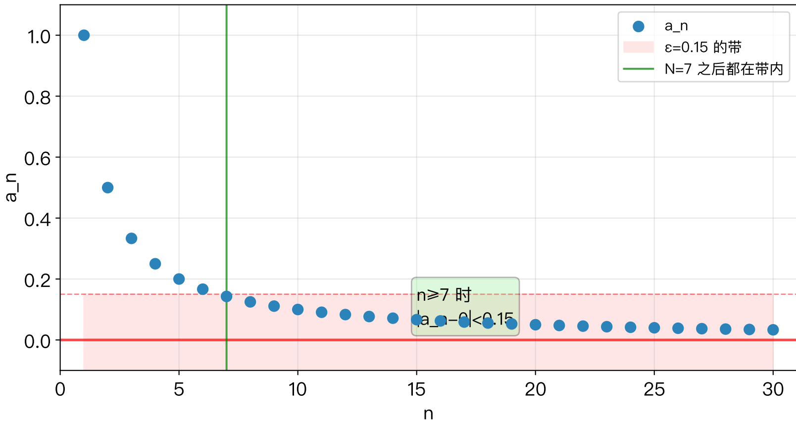
极限的" \varepsilon 带"—— N 之后所有项都在带内
