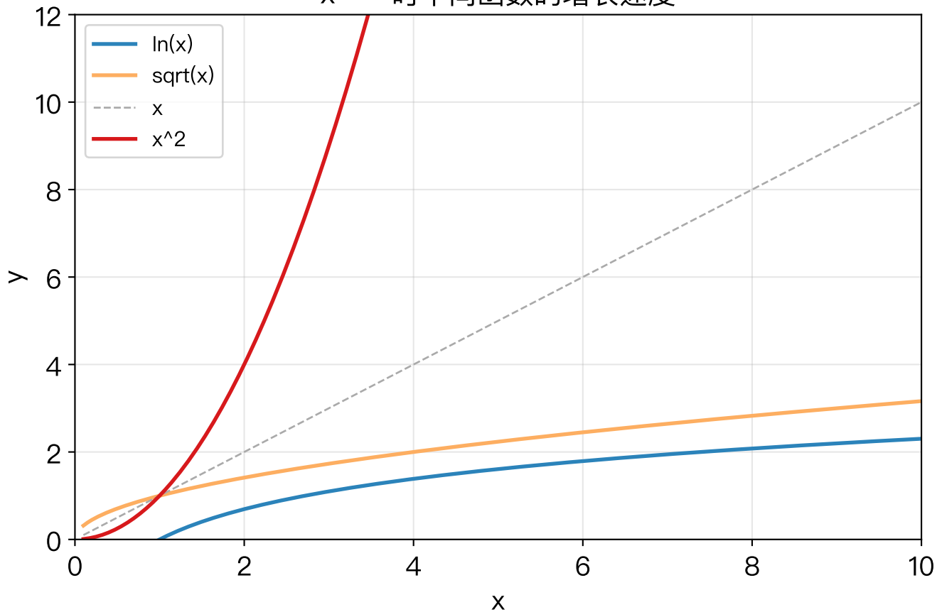
x \rightarrow \infty 时不同函数的增长速度
