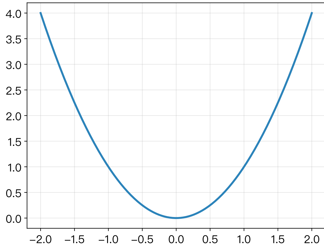
连续函数 —— 一笔画
