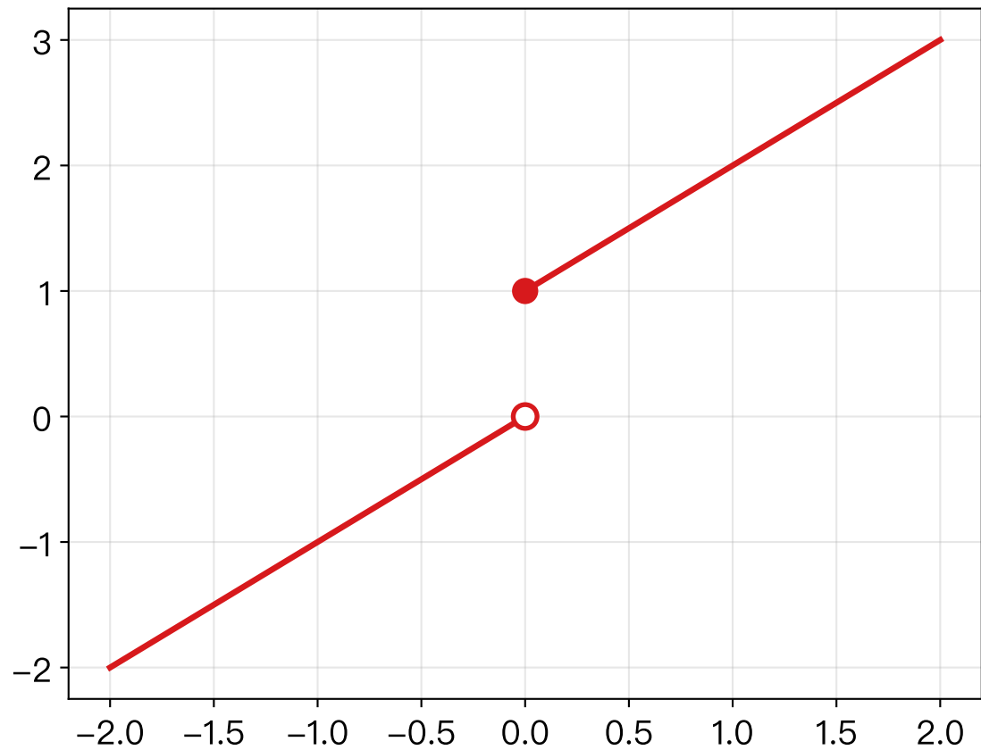
间断函数 —— 笔要断开
