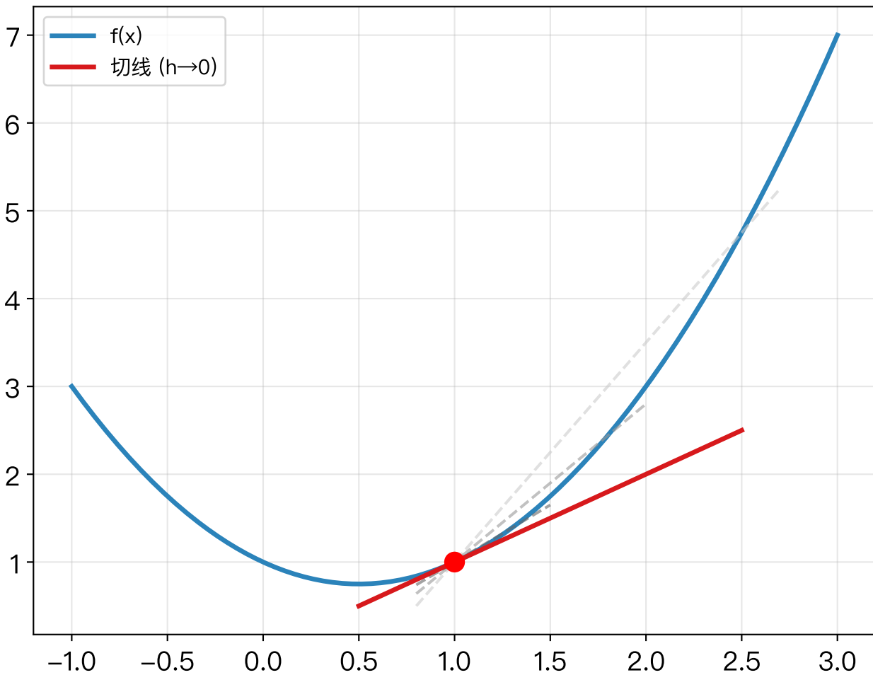
割线→切线： h \rightarrow 0 时割线的极限位置
