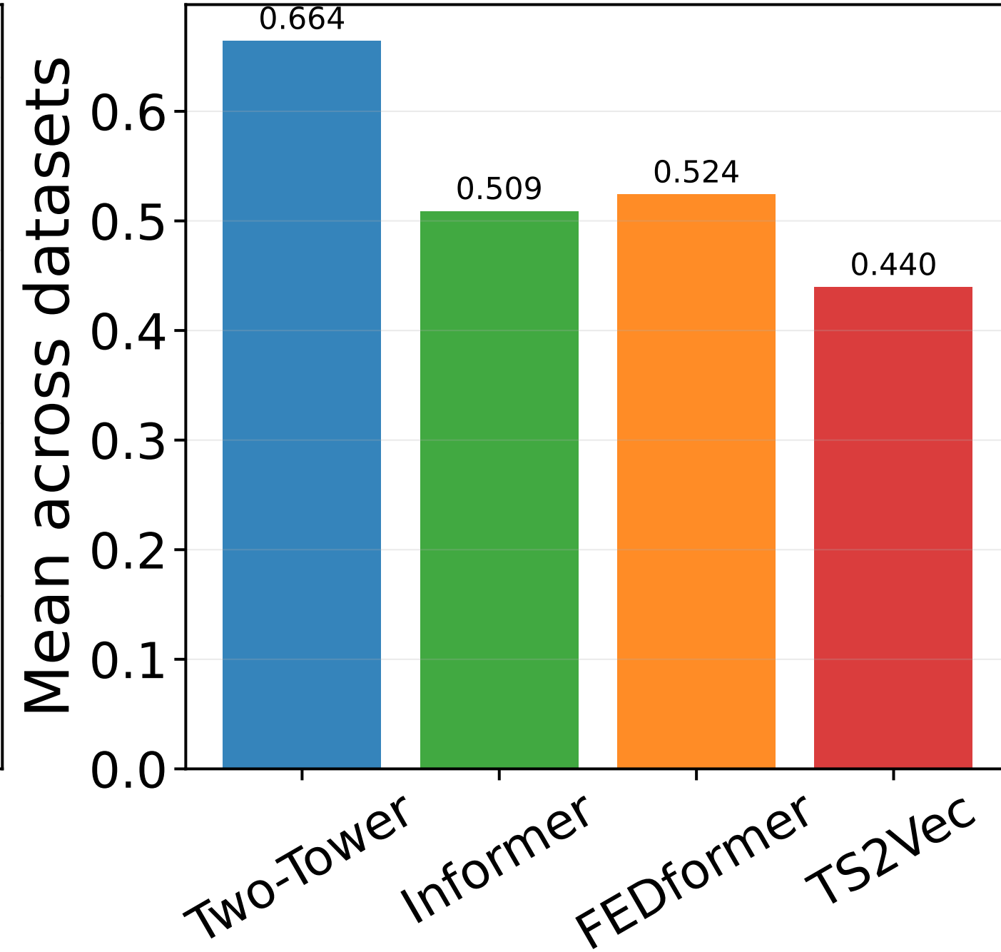
ACC
