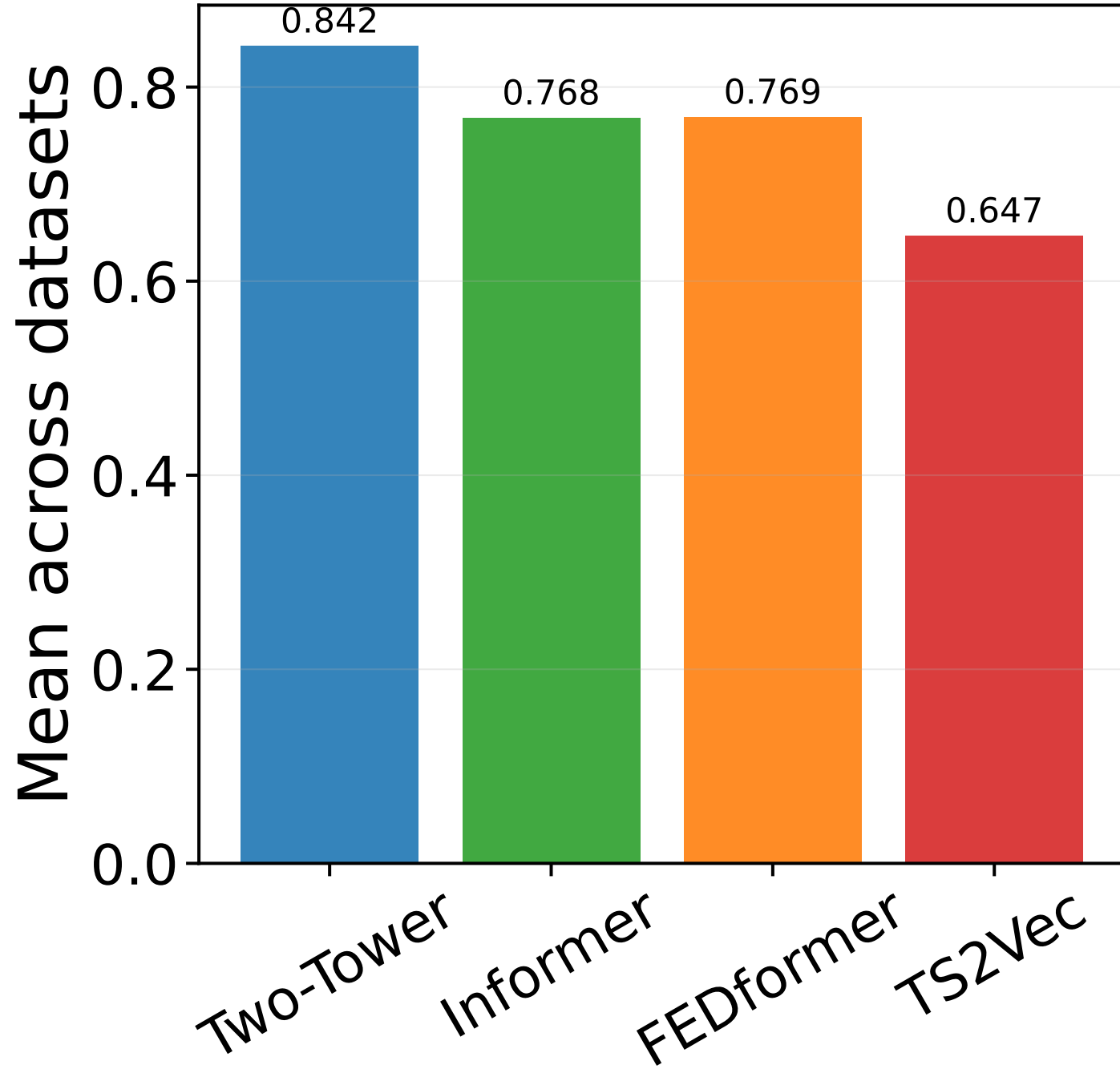
AUC
