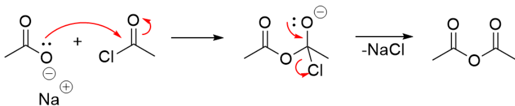
Abbildung 9: Darstellung von Säureanhydriden aus Säurechloriden
