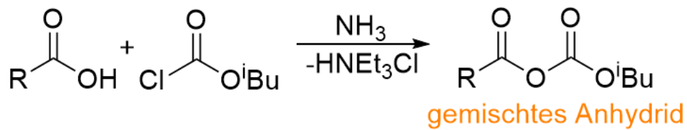
Abbildung 10: Darstellung von gemischten Anhydriden über in situ Aktivierung
