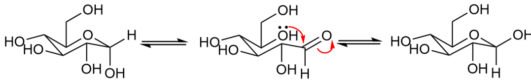
\alpha -Anomeres
