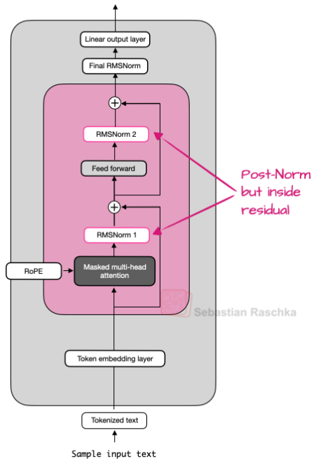
OLMo 2 7B
