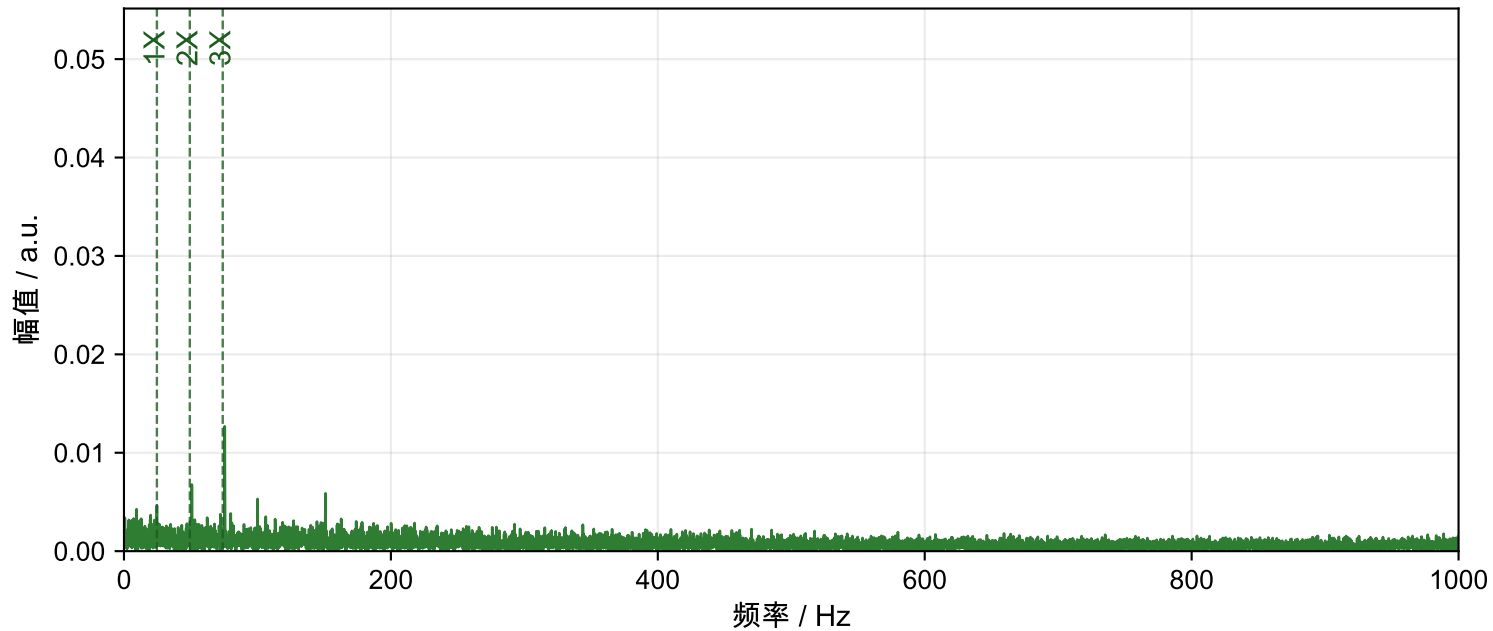
Motor-2 松动 包络谱
