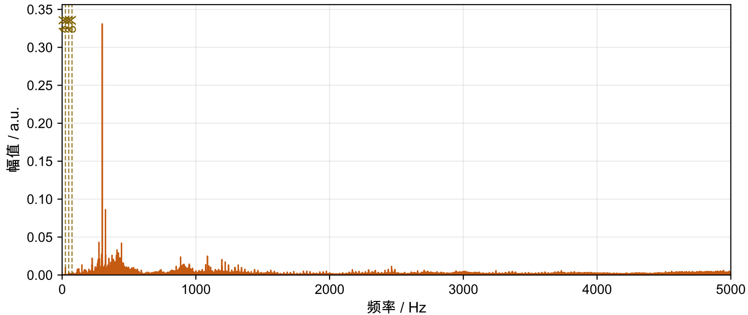
Motor-2 轴承故障 FFT频谱 (5000 Hz)
