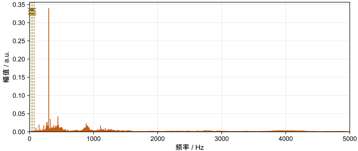
Motor-2 松动 FFT频谱 (5000 Hz)
