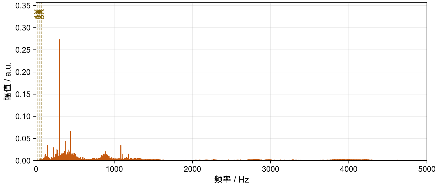
Motor-2 正常 FFT频谱 (5000 Hz)
