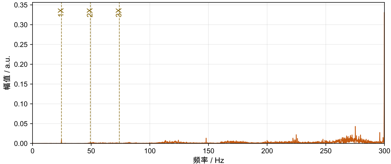
Motor-2 轴承故障 FFT频谱 (300 Hz)
