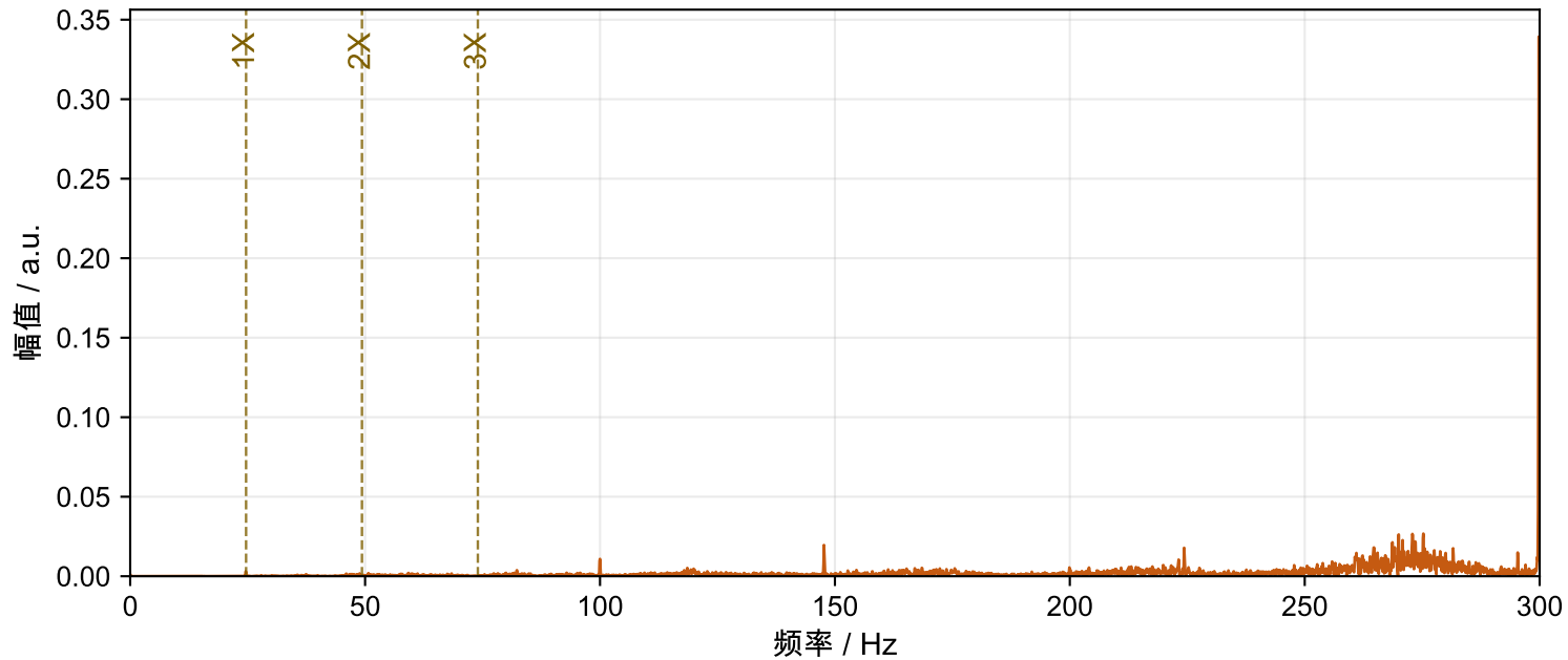
Motor-2 松动 FFT频谱 (300 Hz)
