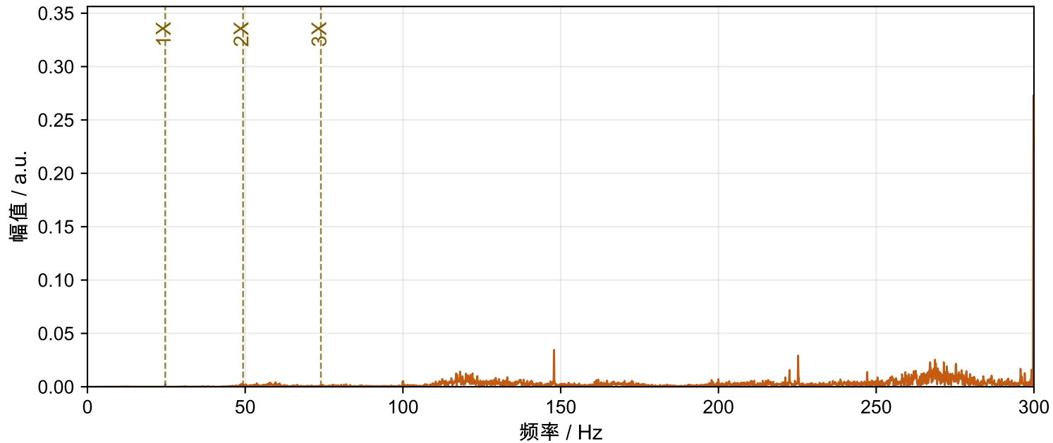
Motor-2 正常 FFT频谱 (300 Hz)
