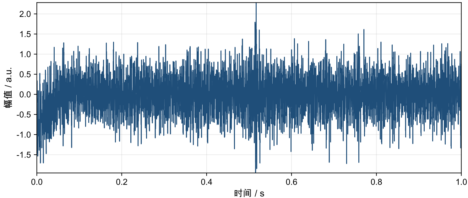
Motor-2 轴承故障 时域波形
