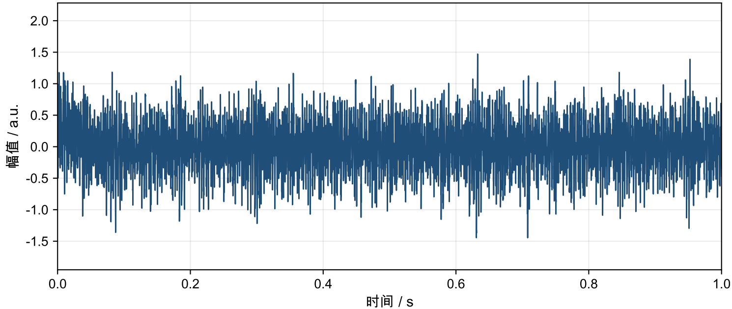
Motor-2 松动 时域波形
