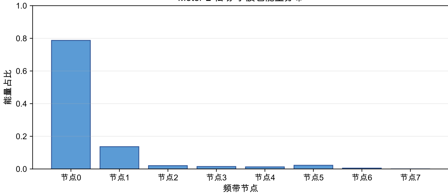
Motor-2 松动 小波包能量分布
