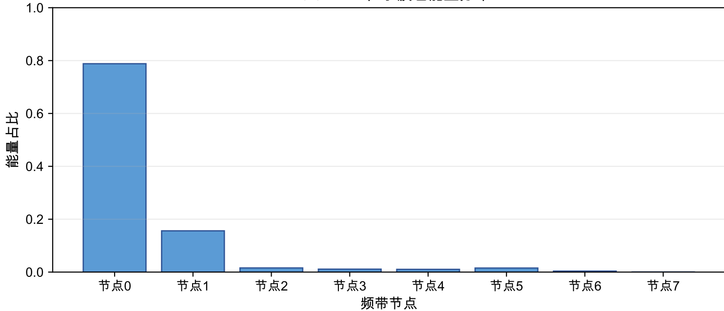
Motor-2 正常 小波包能量分布
