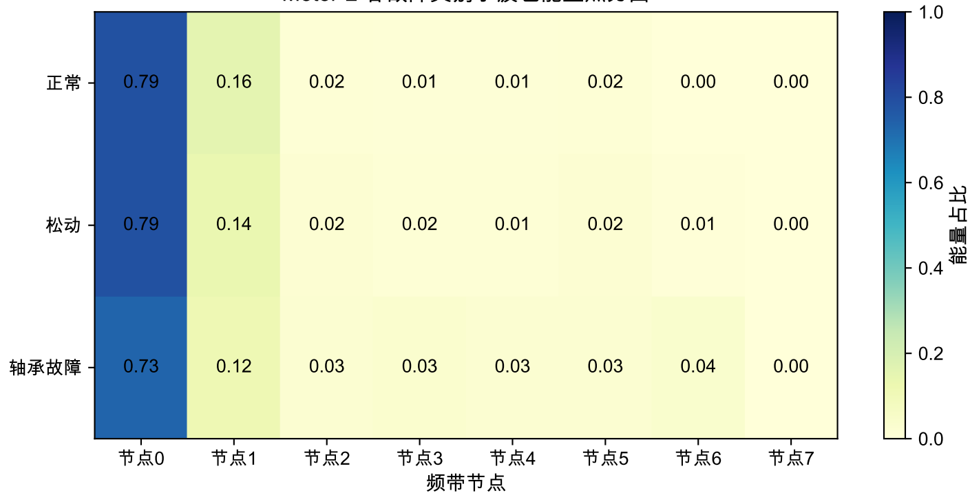
Motor-2 各故障类别小波包能量热力图
