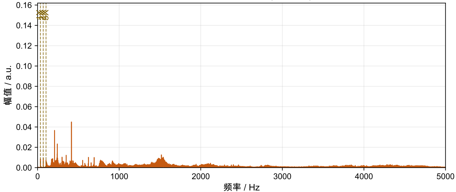
Motor-4 汽蚀 FFT频谱 (5000 Hz)
