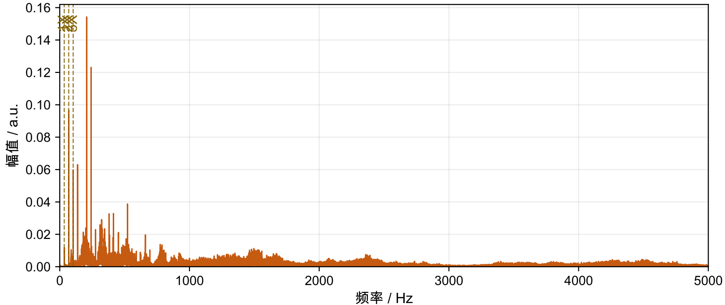
Motor-4 联轴器不对中 FFT频谱 (5000 Hz)
