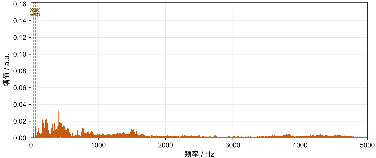
Motor-4 正常 FFT频谱 (5000 Hz)
