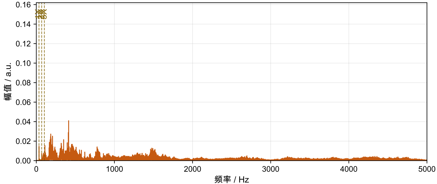
Motor-4 转子不平衡 FFT频谱 (5000 Hz)
