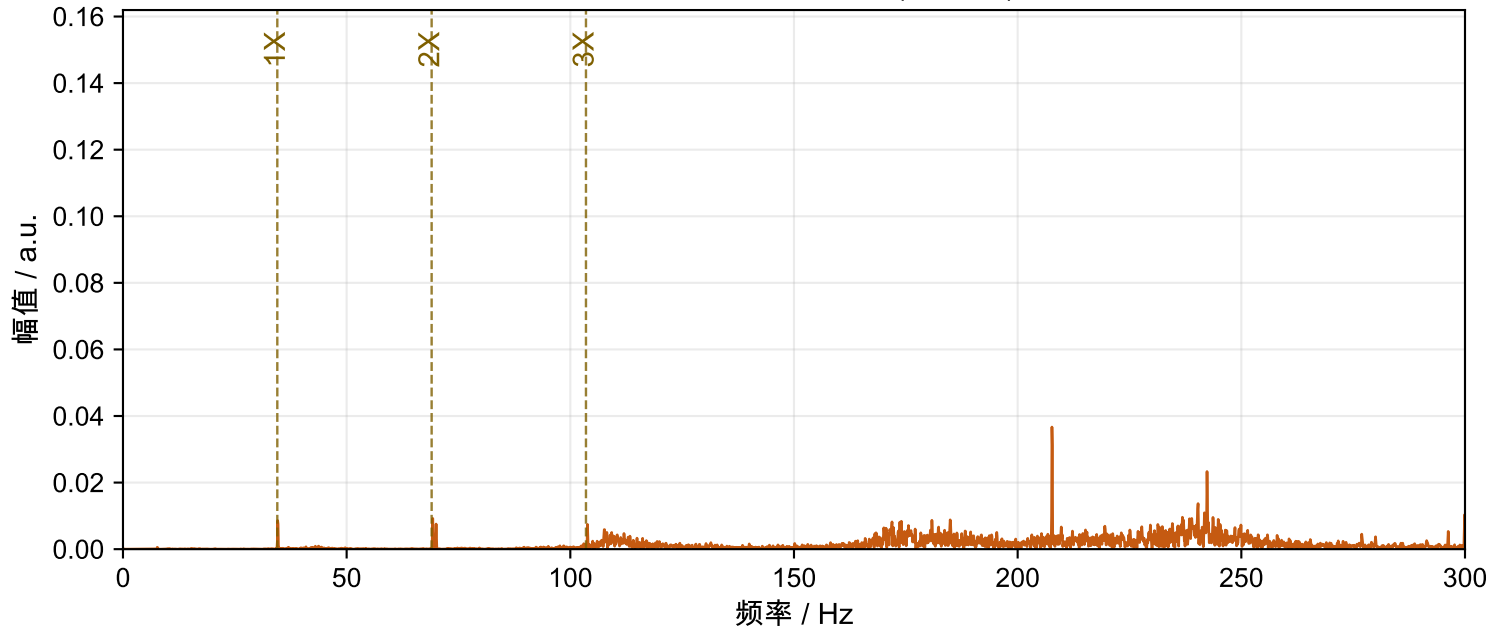
Motor-4 汽蚀 FFT频谱 (300 Hz)
