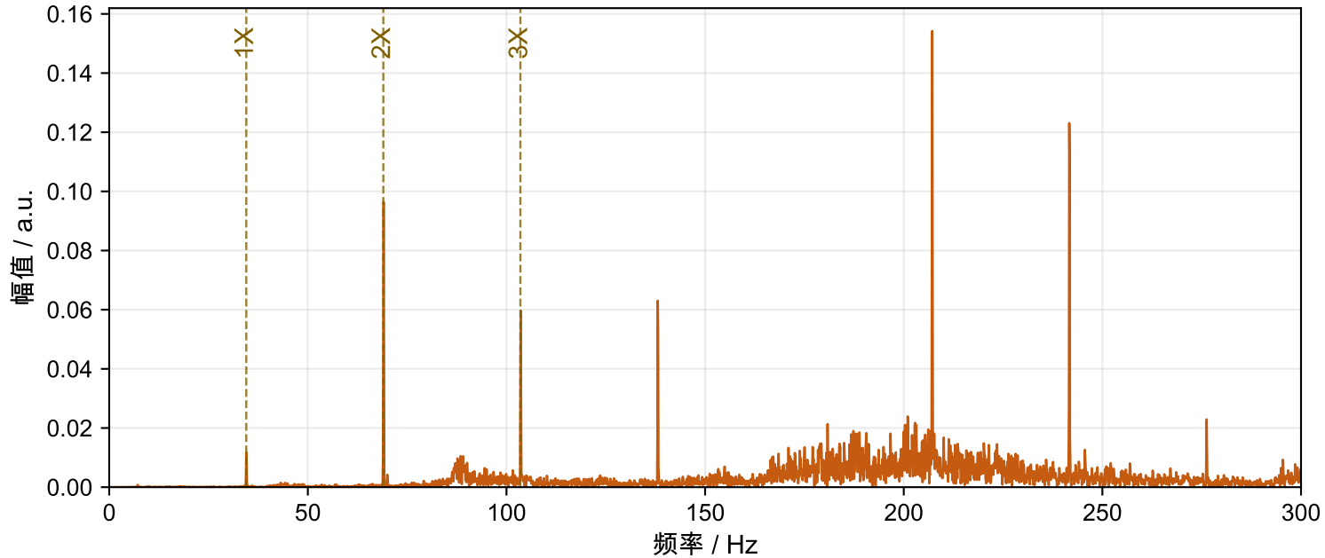
Motor-4 联轴器不对中 FFT频谱 (300 Hz)
