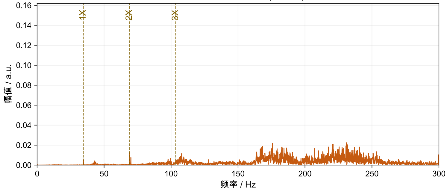
Motor-4 正常 FFT频谱 (300 Hz)
