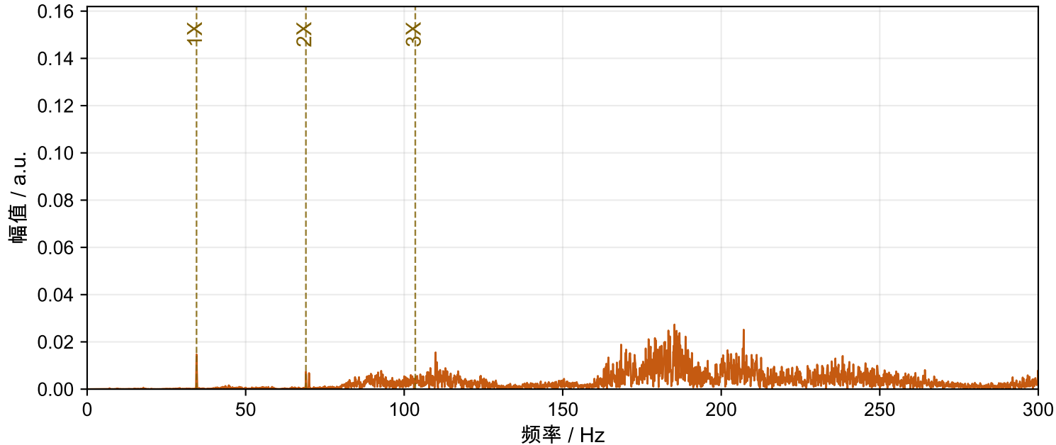
Motor-4 转子不平衡 FFT频谱 (300 Hz)
