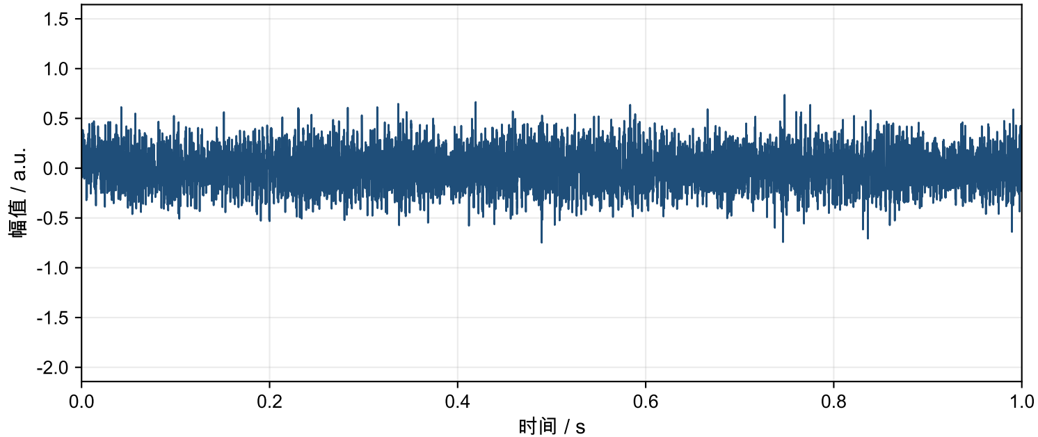
Motor-4 汽蚀 时域波形
