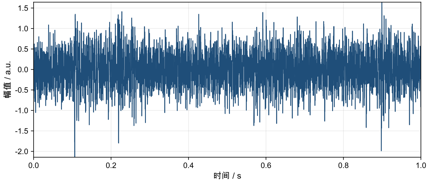
Motor-4 联轴器不对中 时域波形
