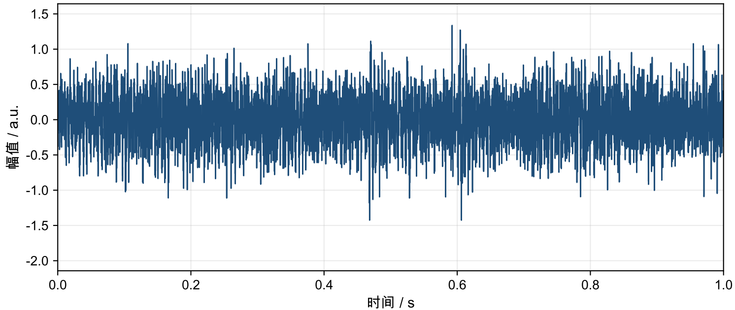
Motor-4 转子不平衡 时域波形
