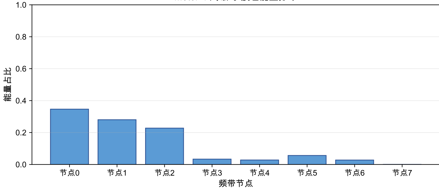
Motor-4 汽蚀 小波包能量分布
