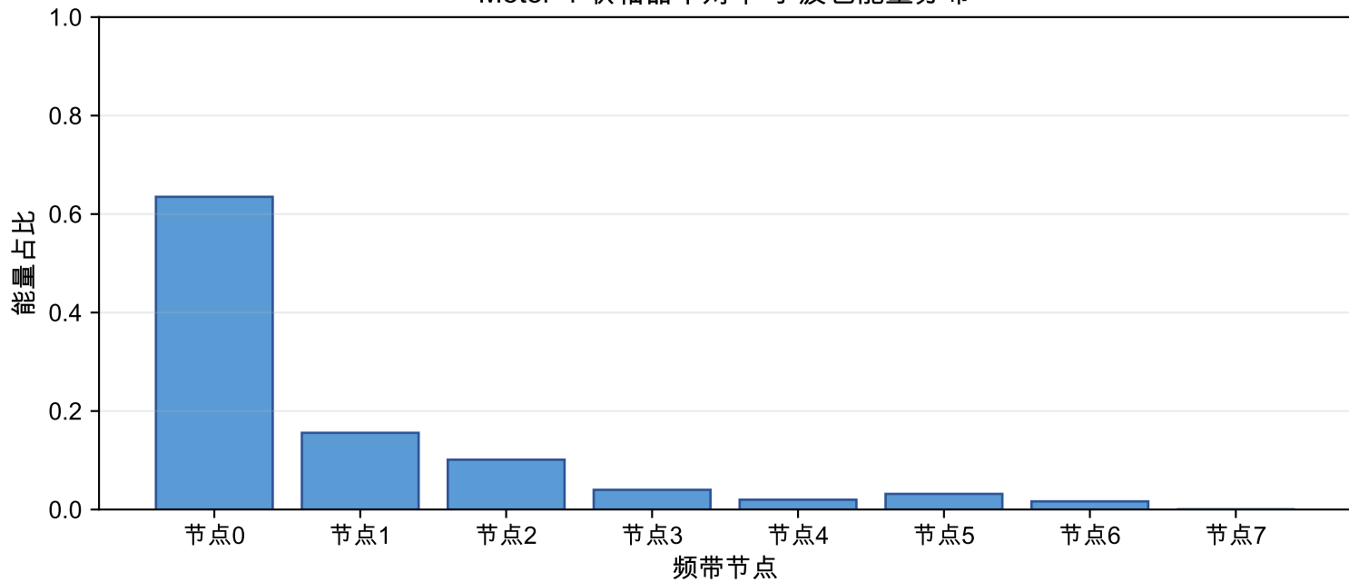
Motor-4 联轴器不对中 小波包能量分布
