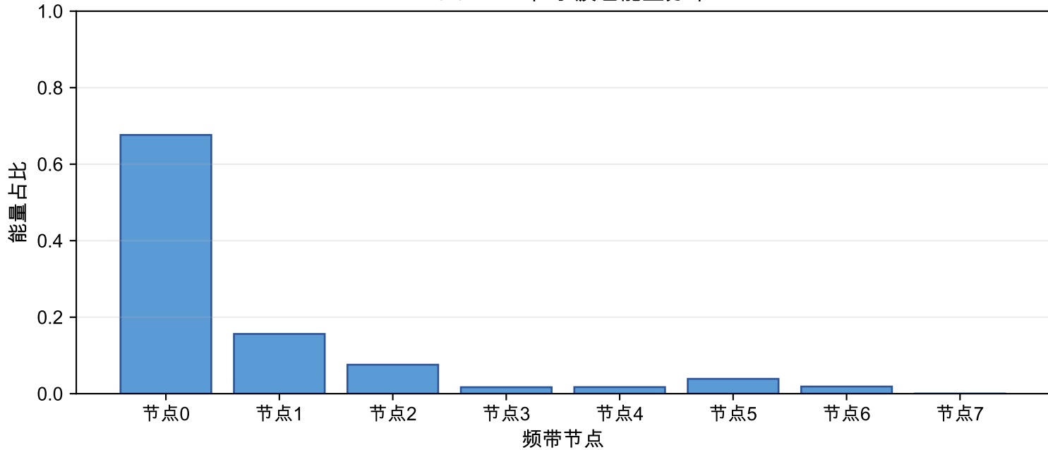
Motor-4 正常 小波包能量分布
