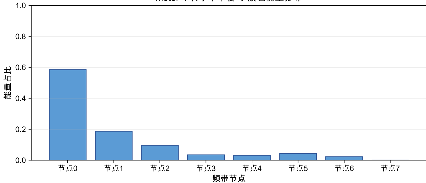
Motor-4 转子不平衡 小波包能量分布
