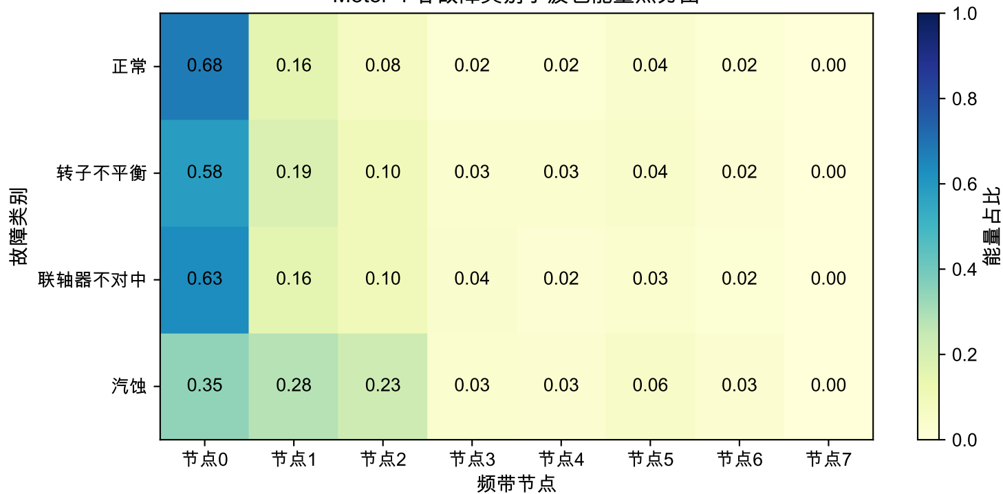
Motor-4 各故障类别小波包能量热力图
