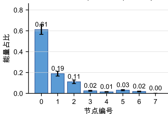
联轴器不对中 | Motor-4 | 2070 rpm
