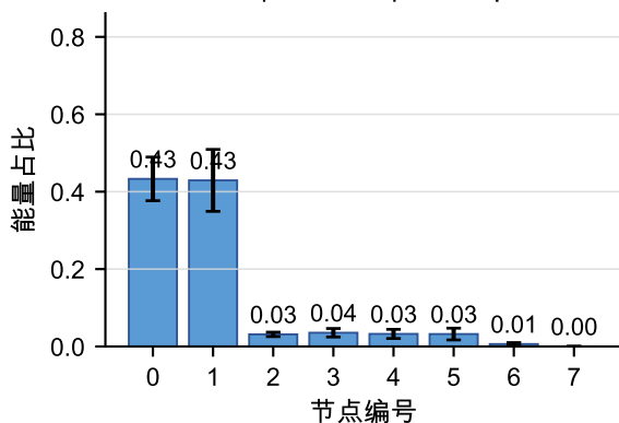
松动 | Motor-2 | 1110 rpm
