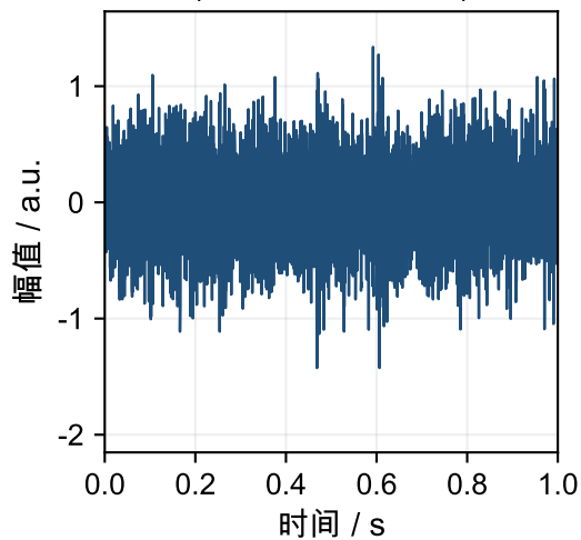
转子不平衡 (70%, 2070 r/min)
