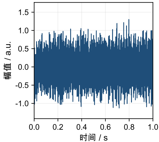
转子不平衡 (70%, 2070 r/min)
