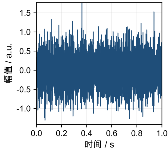
联轴器不对中 (70%, 2070 r/min)
