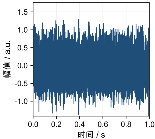
正常 (70%, 2070 r/min)
