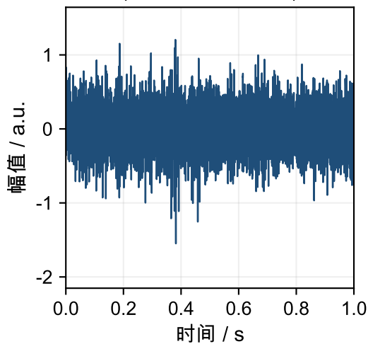
正常 (70%, 2070 r/min)
