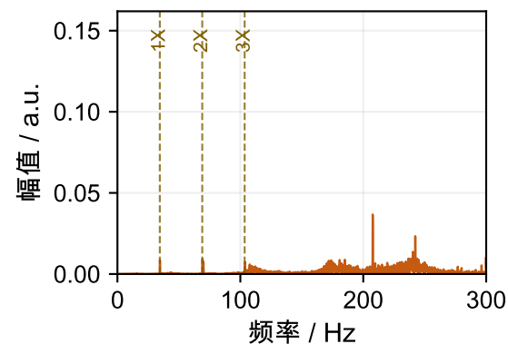
汽蚀 (70%, 2070 r/min) 低频
