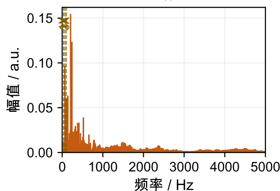
联轴器不对中 (70%, 2070 r/min) 全频
