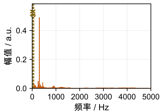
转子不平衡 (70%, 2070 r/min) 全频
