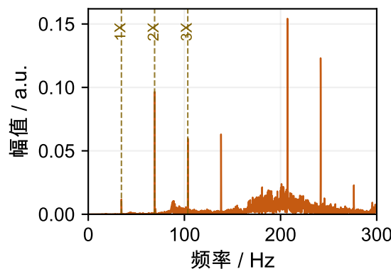
轴承故障 (100%, 1480 r/min) 全频
