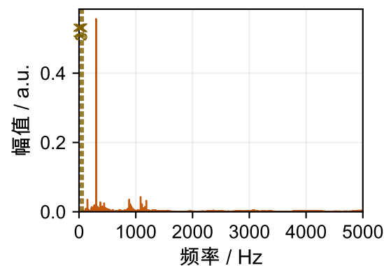
正常 (70%, 2070 r/min) 全频
