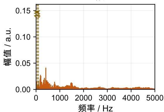
转子不平衡 (70%, 2070 r/min) 全频
