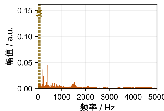
汽蚀 (70%, 2070 r/min) 全频
