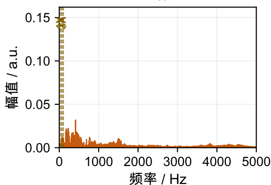
正常 (70%, 2070 r/min) 全频
