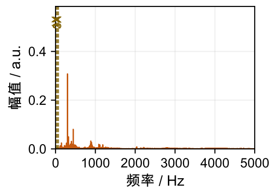
联轴器不对中 (70%, 2070 r/min) 全频
