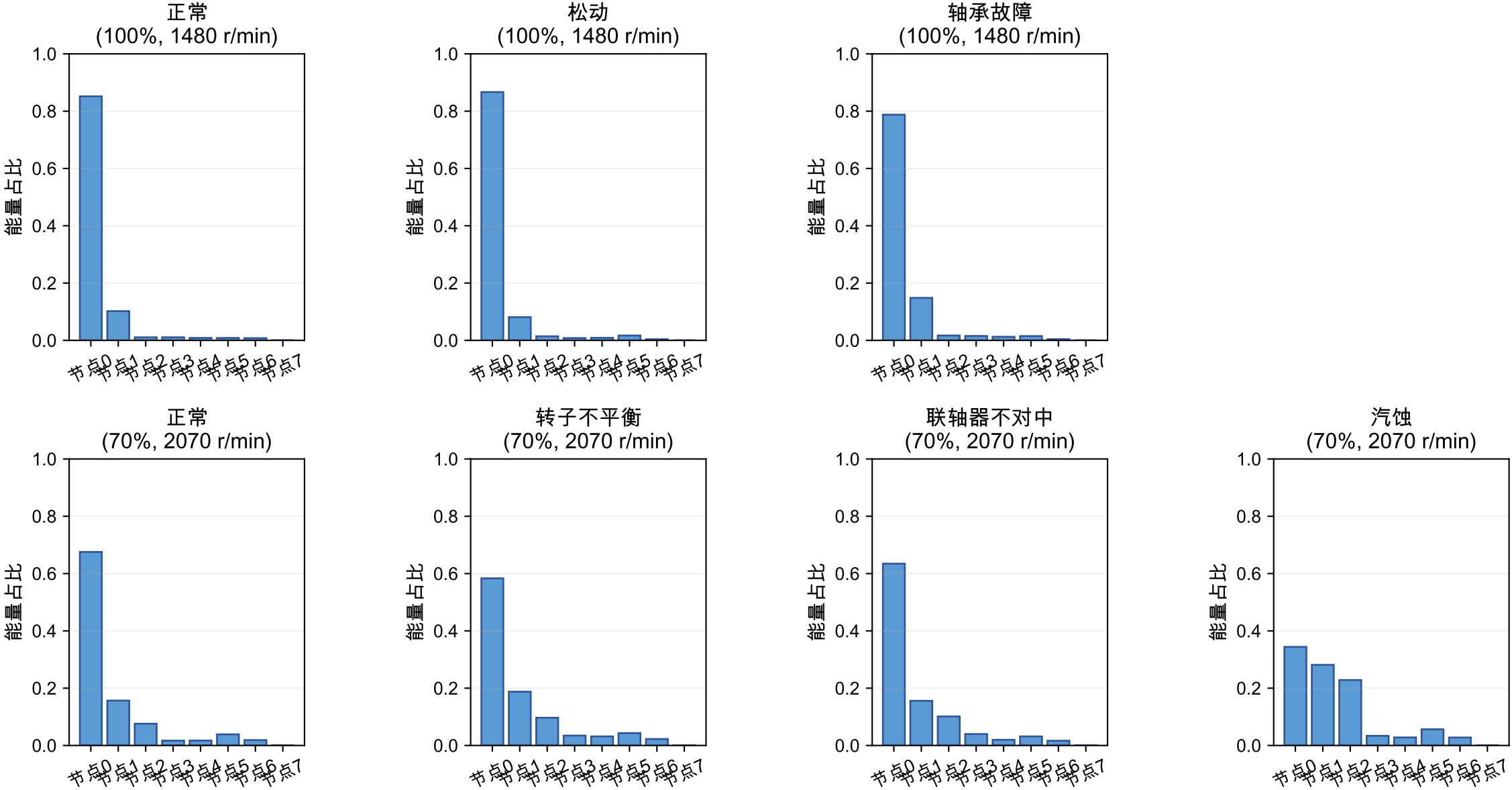
代表样本小波包能量分布
