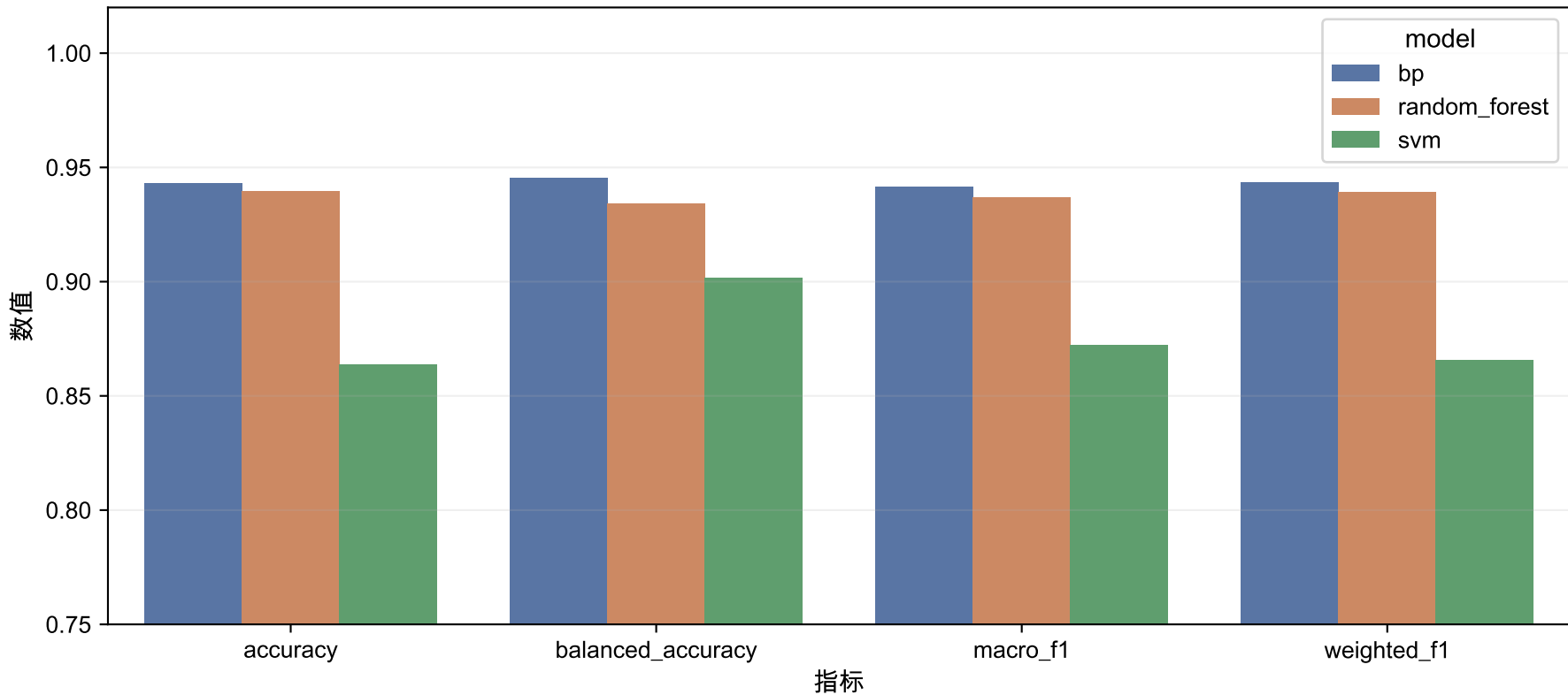
三种模型窗口级指标对比
