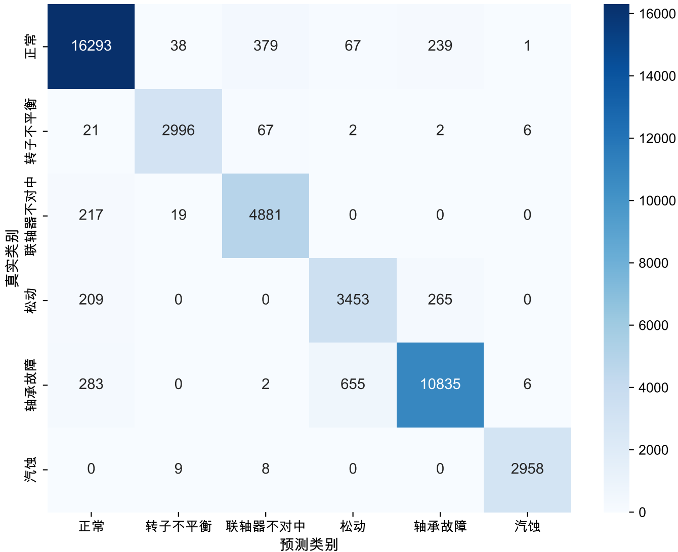
BP神经网络测试集混淆矩阵
