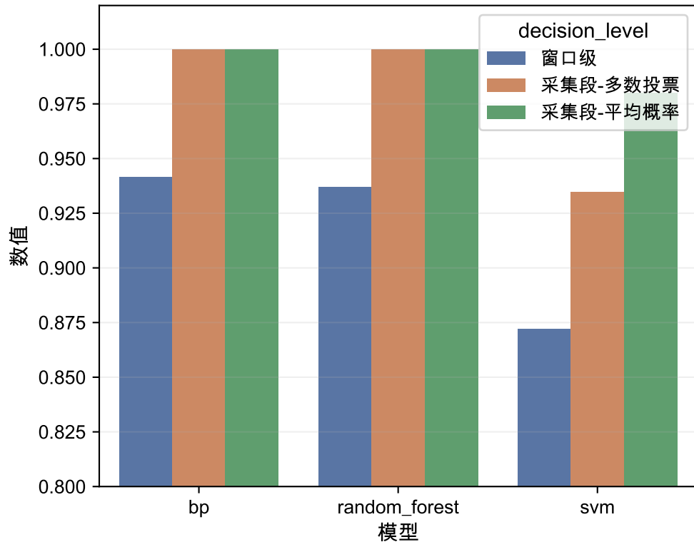
Macro-F1 对比
