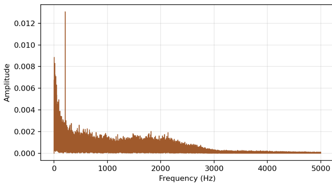
图：包络谱
