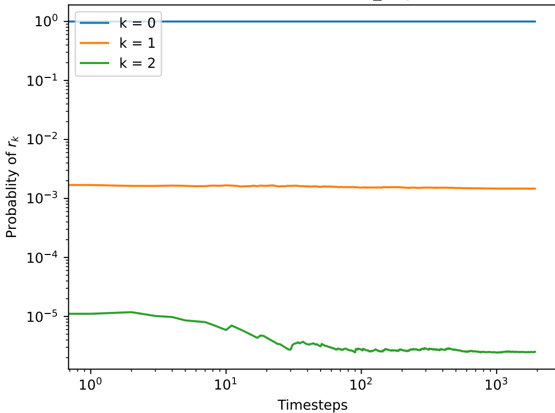
threads-ask-ubuntu_orig
